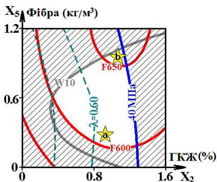
Рис.2. Приклад вибору оптимальних складів суднобудівних керамзитобетонів (кількість портландцементу 600 \text{ кг/м}^3 , добавки С-3 – 0.8%, добавки Пенетрон А – 2%)
