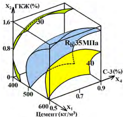
Рис.1 – Вплив кількості портландцементу, С-3 і концентрації кремній-органічного гідрофобізатору на міцність при стиску суднобудівного керамзитобетону у водонасиченому стані ( x_3=x_5=0 ).
