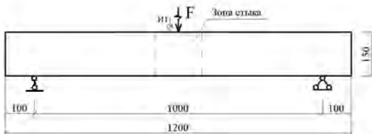
Рис.3. Схема динамического испытания образцов балок ( F -амплитуда динамической силы вибромашины; И1-акселерометр)
