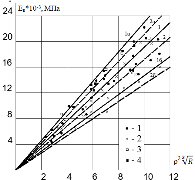
Рис.3. Зависимость модуля упругости керамзитобетона от \rho^2\sqrt[3]{R} : 1- керамзитобетон на карбонатном песке естественного твердения; 2 - то же, пропаренный; 3- керамзитобетон на кварцевом песке естественного твердения; 4 - то же, пропаренный.
