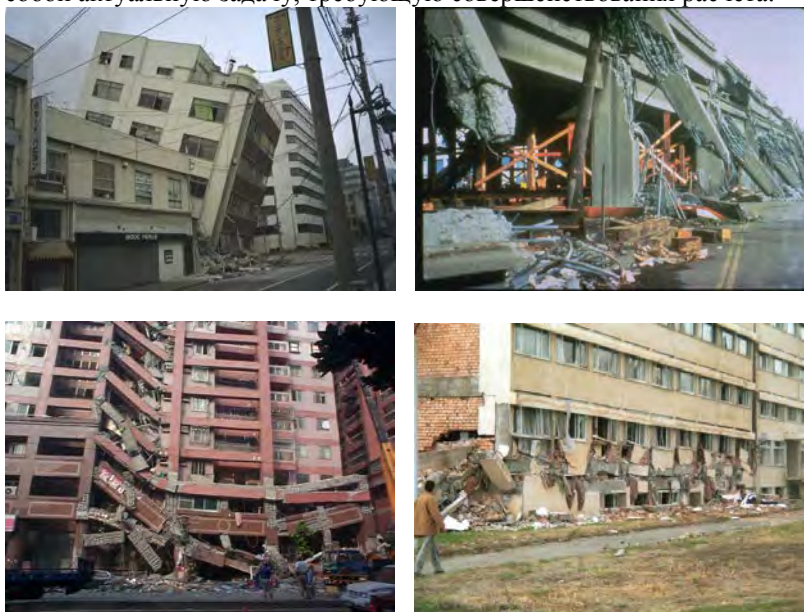
Фото 1-4. Характер разрушения каркасных зданий от сейсмического воздействия
