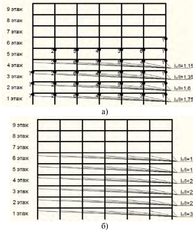
Рис.2 Соотношения жесткостей необходимого усиления с учетом появляющихся пластических деформаций (а) и без учета таковых (б) в продольном направлении расчетной схемы
