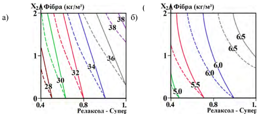
Рис.2. Вплив кількості фібри і пластифікатору на міцність піщаного бетону (а) – при стиску; (б) – на розтяг при згині; ---- гідрофобізоване волокно, ——— контроль
