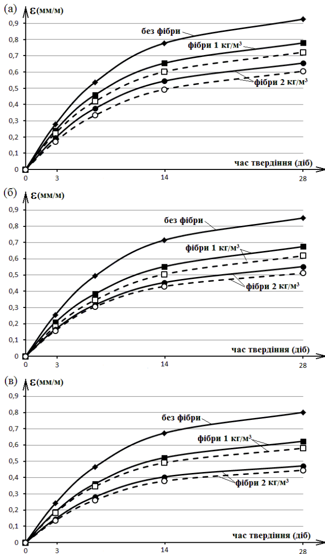
Рис.3. Лінійна усадка досліджених піщаних бетонів. Кількість добавки Релаксол Супер ПК: а) – 0.4%, б) – 0.8%, в) – 1.2%. - - - - гідрофобізоване волокно, — контроль
