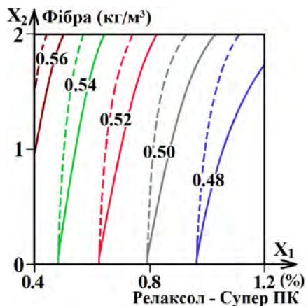
Рис.1. Вплив кількості фібри і пластифікатору на В/Ц сумішей рівної рухомості. ---- гідрофобізоване волокно, — контроль.
