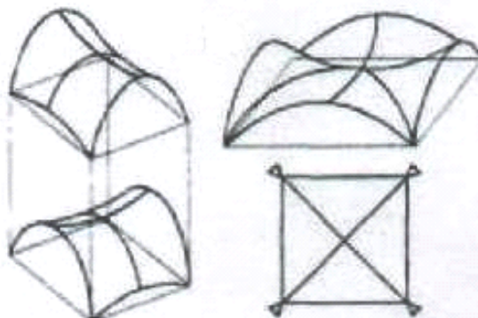
Рис. 2. Схемы покрытий из гипаров с криволинейным контуром.
