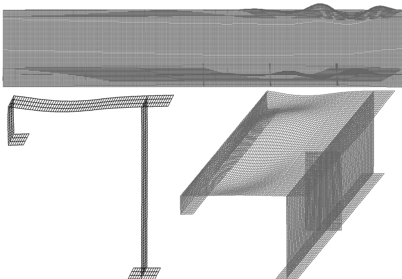
Рис. 9. Форма местной потери устойчивости листа тормозной балки: вид сверху, поперечное сечение, фрагмент конструкции
