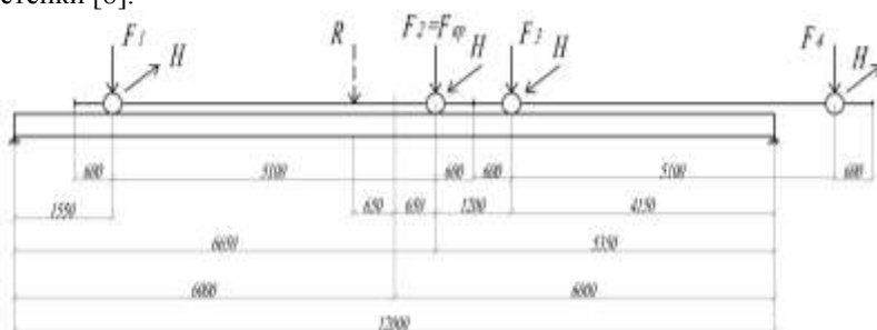
Рис. 3. Размещение системы вертикальных грузов на балке по теореме Винклера
