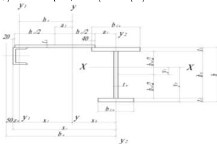
Рис. 1. Поперечное сечение подкрановой балки с тормозной балкой
