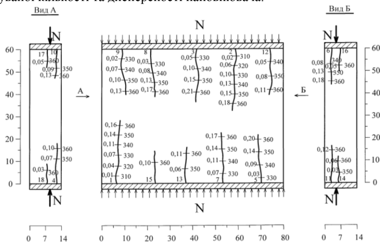
Рис. 1. Узагальнена схема руйнування моделей стінових елементів СП-1 А ... СП-11 А , з шириною розкриття тріщин \alpha^{cr} (мм) та навантаженням (кН) для СП-2 Б .
