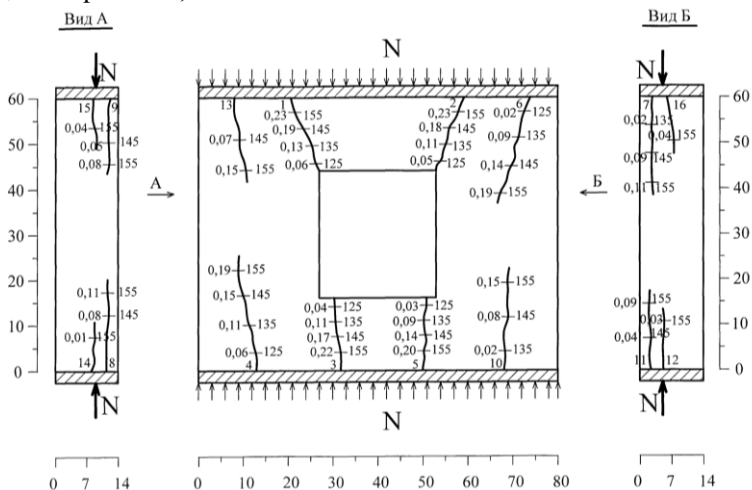
Рис. 2. Узагальнена схема руйнування моделей стінових елементів СП-2'А... СП-4'А, СП-2'Б... СП-4'Б, з шириною розкриття тріщин a^{crc} (мм) та навантаженням (кН) для СП2'А.
