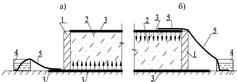
Рис. 2. Схемы капиллярного увлажнения: а) поднятого; б) подвешенного. 1 - кольцо прибора; 2 - образец грунта; 3 - хлопчатобумажная ткань (фильтровальная бумага); 4 - емкость с водой; 5 - фитиль из хлопчатобумажной ткани
