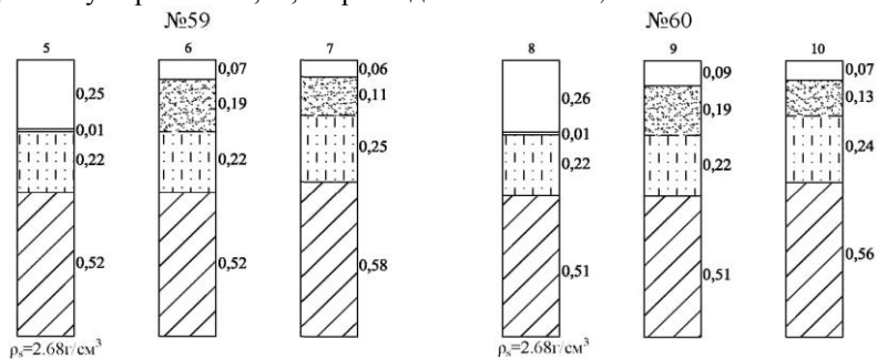
Рис. 4. Изменения емкостей фаз и фазовых компонентов под влиянием внешней нагрузки при капиллярно–поднятом увлажнении
