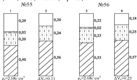
Рис. 3. Изменение емкостей фаз и фазовых компонентов в грунтах природной влажности под влиянием внешней нагрузки
