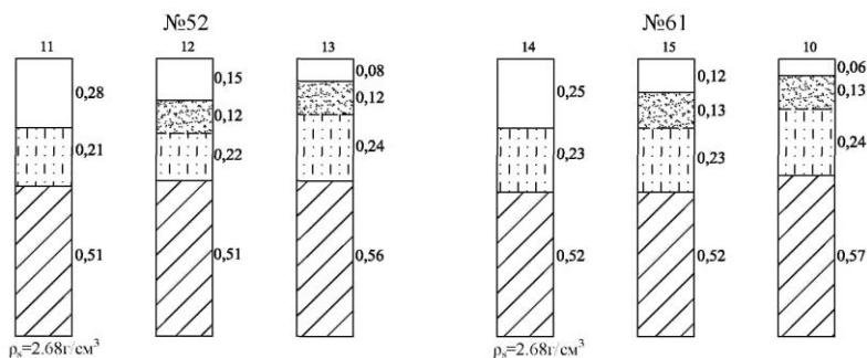
Рис. 5. Изменение емкостей фаз и фазовых компонентов под влиянием внешней нагрузки при капиллярно–подвешенном увлажнении
