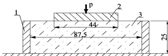
Рис. 1. Схема прибора для испытаний с возможностью поперечных деформаций. Размеры в мм. 1 - кольцо прибора; 2 - штамп; 3- образец грунта
