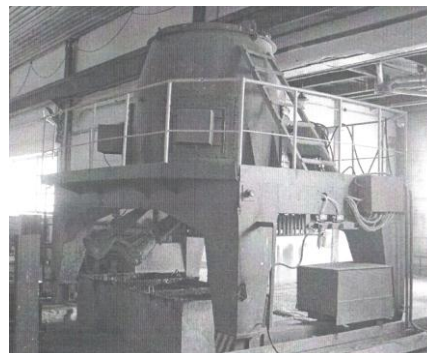
Рис.4. Виброгазобетономешалка по приготовлению растворной смеси
