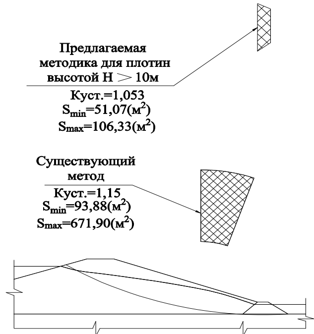
Рис. 4. Области расположения кривых обрушения с минимальным значением коэффициента запаса на устойчивость. Для плотин высотой 10 м–25 м
