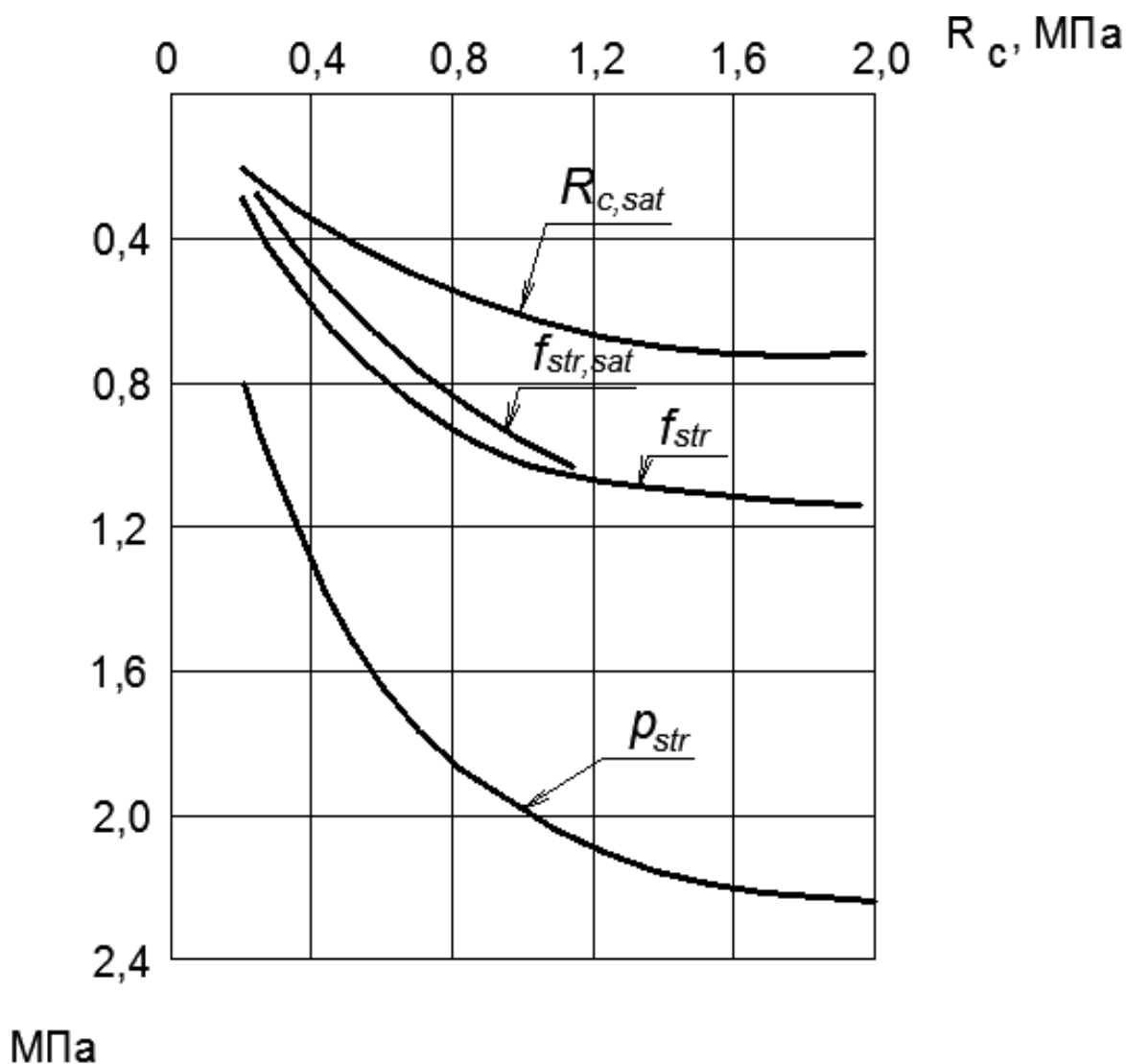
Рис.1. Корреляционные зависимости предельных значений параметров прочностных свойств пыльного известняка-ракушечника от предельной прочности на одноосное сжатие
