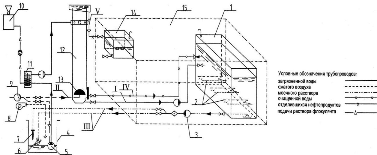
Рис. 1. Принципиальная схема мобильной флокуляционно-флотационной установки для очистки промывных нефтесодержащих сточных вод:
