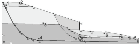
Рис. 6. Размещение точек получения анализируемых акселерограмм
