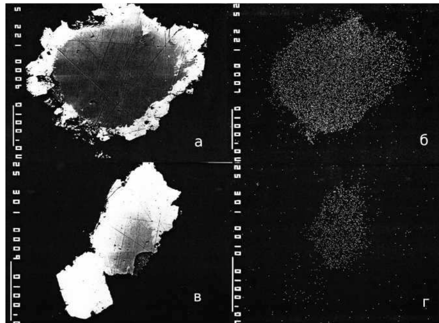
Рис. 1. Рентгенівські знімки зонального золота з донних відкладів району Тендрівської коси у вторинних електронах (а, в) та ті ж зразки в характерному випромінюванні по лінії La Ag (б, г), масштабна мітка відповідає 0,1 мм
