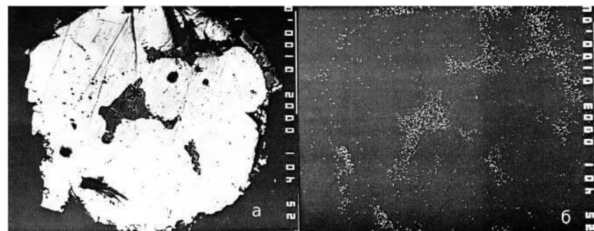
Рис. 2. Рентгенівський знімок зонального золота з донних відкладів району Затоки у вторинних електронах (а) та в характерному випромінюванні по лінії La Pb (б), масштабна мітка відповідає 0,1 мм
