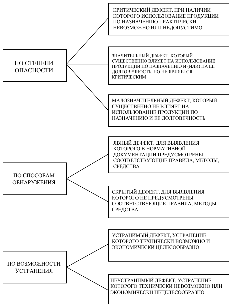
Рис. 1. Классификация дефектов
