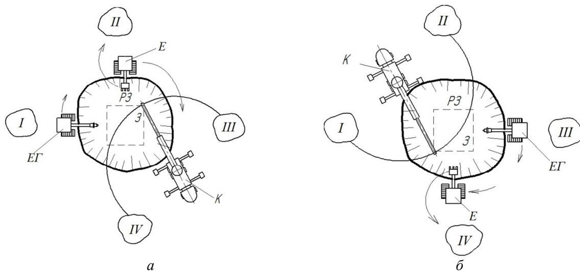
Рис. 4. Схема розстановки і переміщення техніки при розбиранні поширених завалів зруйнованої будівлі: а – початковий етап; б – закінчення розбирання завалу. ЕГ – однокішований екскаватор ыз гідромолотом; Е – однокішований екскаватор; К – автокран з гаковою підвіскою або захватом; I – IV – майданчики-відвали. З – будівля; РЗ – зруйнована будівля
