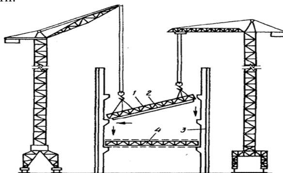
Рис. 1. Монтаж тяжёлых конструкций двумя башенными кранами: 1 – монтажная ферма, 2 – усиление нижнего пояса фермы, 3 – опоры, 4 – смонтированная ферма
