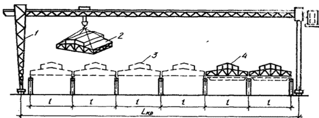
Рис. 3. Схема установки козловых кранов при методе монтажа покрытий реконструируемого дока:
