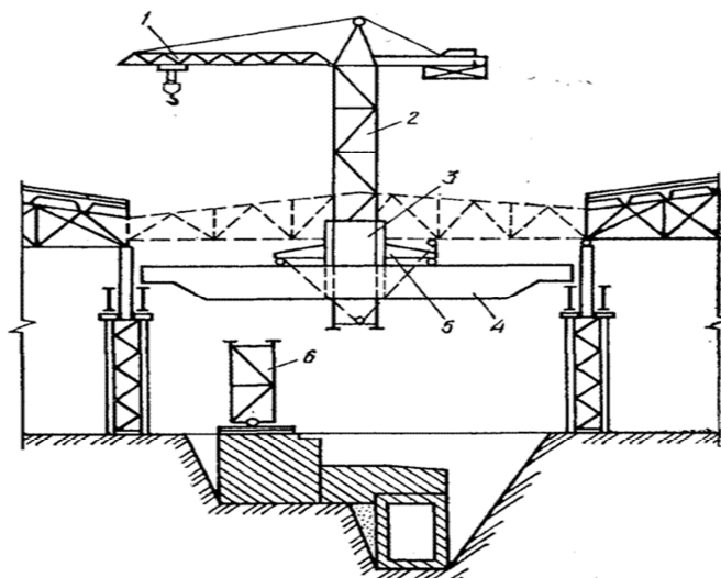
Рис. 2. Схема использования мостового крана со сменной башенно-стреловой оснасткой: 1 – полноповоротная стрела, 2 – башня, 3 – обойма, 4 – электромостовой кран, 5 – тележка; 6 – секция башни
