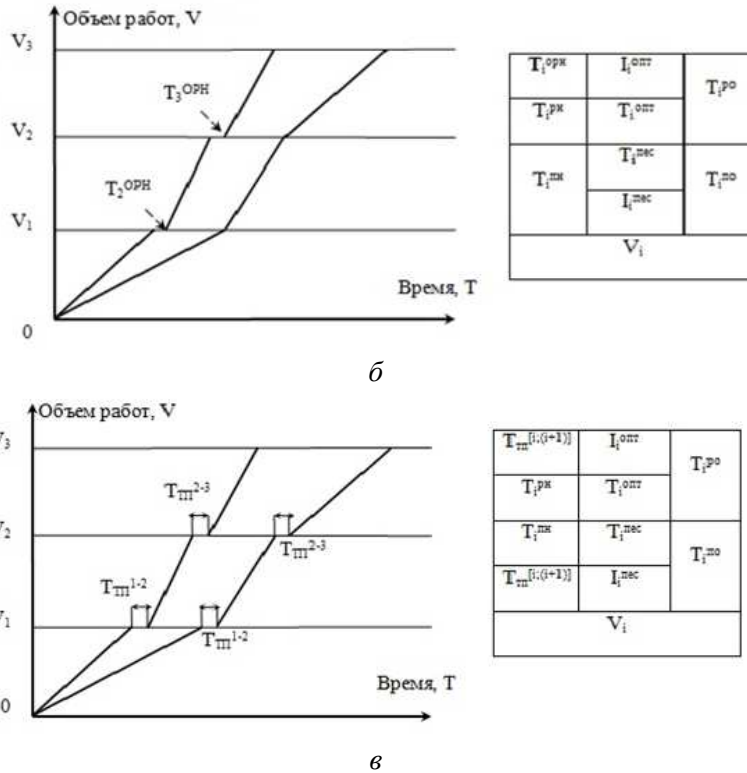
Рис. 1. Циклограммы возможных вариантов выполнения последовательных этапов одной работы и соответствующие им квадраты (матрицы) расчетных временных параметров; а – выполнение работ без дополнительных ограничений; б – выполнение работ с ограничениями по ранним началам; в – выполнение работ с технологическими перерывами между смежными этапами
