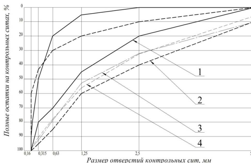
Рис. 1. Соотношение зерновых составов шлаков и рекомендуемого зернового состава заполнителей для бетонов: 1 – область рекомендованного зернового состава заполнителя для тяжелого бетона; 2 – область рекомендованного зернового состава заполнителя для конструктивно-теплоизоляционного легкого бетона; 3 – кривая зернового состава доменного гранулированного шлака ПАО «ЕВРАЗ-ДМЗ им.Петровского»; 4 – кривая зернового состава гранулированного шлака силикомарганца ПАО «Никопольский завод ферросплавов»
