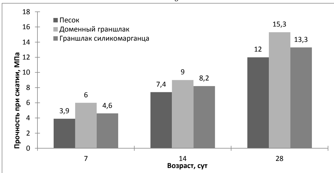
Рис. 2. Результаты лабораторных исследований мелкозернистого бетона на основе разных заполнителей: а – соотношение цемент / заполнитель = 1 : 3, В/Ц = 0,65;
