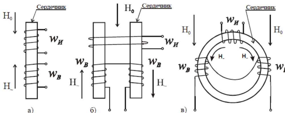
Рис. 1. Варианты конструкций феррозондов:
