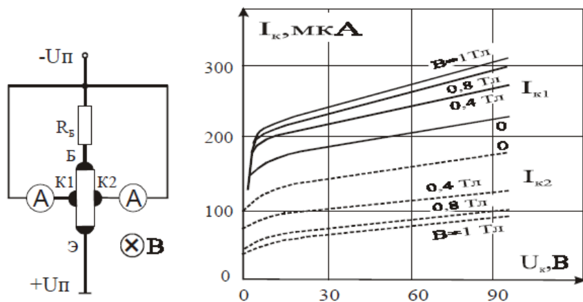
а Рис. 5. Торцевой германиевый двухколлекторный магнитотранзистор: а – структура; б – статические выходные характеристики
