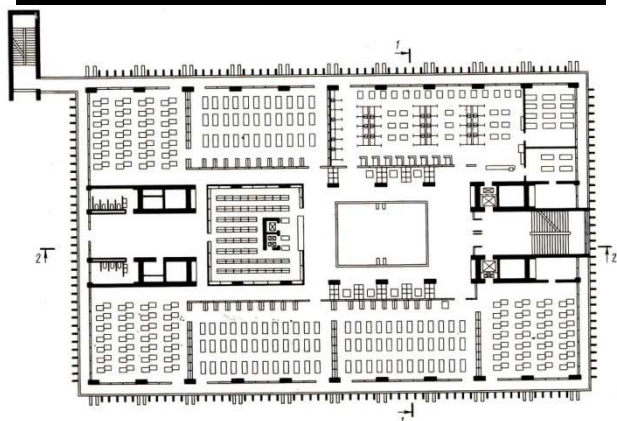
Рис. 7. Днепропетровская межвузовская научная библиотека. Фото с макета и план типового этажа
