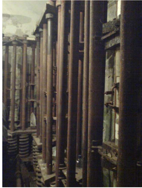
Рис. 4. Пружинні пристрої для тривалих випробувань призм
