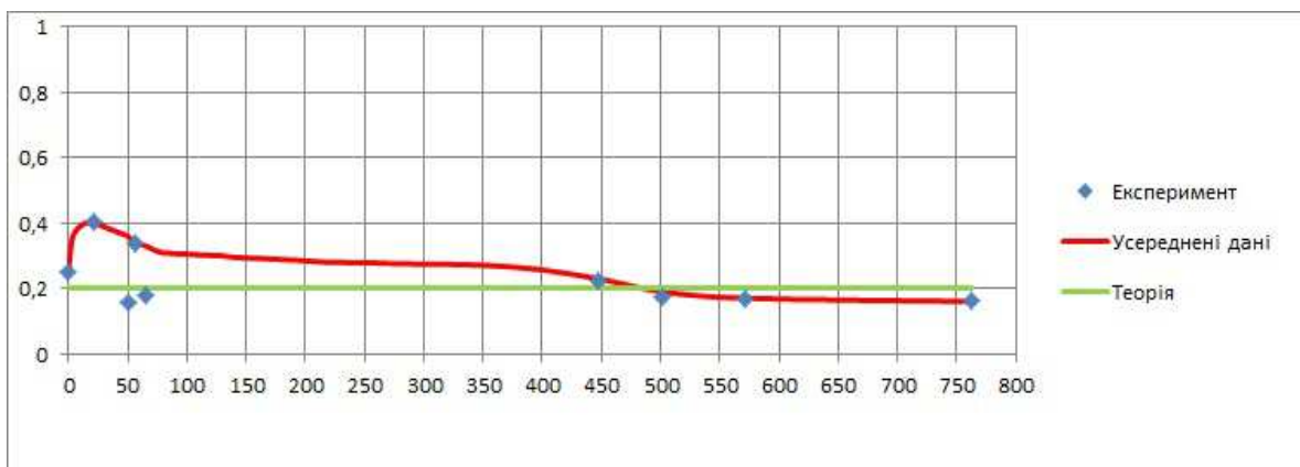
Рис. 7. Графік зміни коефіцієнта повних поперечних деформацій \nu(t) у часі. Вік бетону до моменту навантаження: \tau_1 = 70 діб
