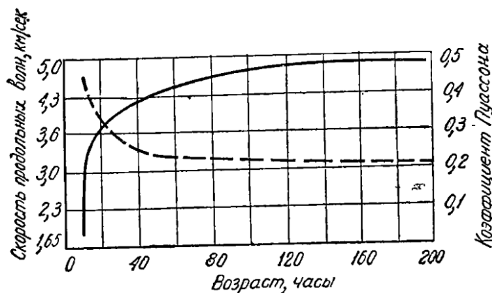
Рис. 1. Зміна швидкості поздовжніх хвиль і коефіцієнта Пуассона з віком бетону [8]
