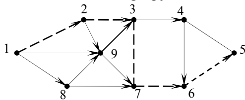
Рис. 2. Граф G_2
