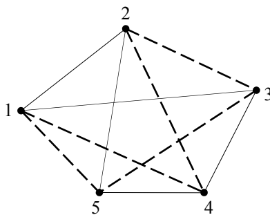
Рис. 3. Граф G_3
