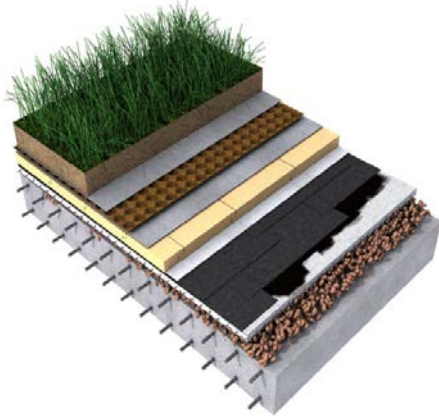
Рис. 7. «Зелёная» кровля
