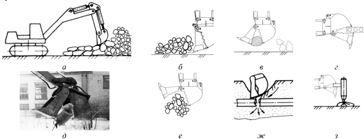
Рис. 4. Використання багатоцільового обладнання (БЦО) на базі екскаваторів: а, б – розроблення дрібних уламків; в, г, д – схоплення великих уламків; е – розвантаження уламків; ж – відновлення інженерних мереж; з – подрібнювання великогабаритних уламків гідромолотом
