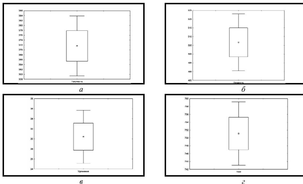
Рис. 2. Гистограммы типа «ящик»: а – предела текучести; б – предела прочности; в – относительного удлинения; г – температура конца прокатки
