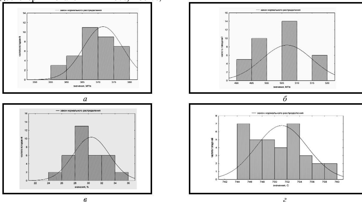
Рис. 1. Гистограммы распределения исследуемых величин: а – предела текучести; б – предела прочности; в – относительного удлинения; г – температура конца прокатки
