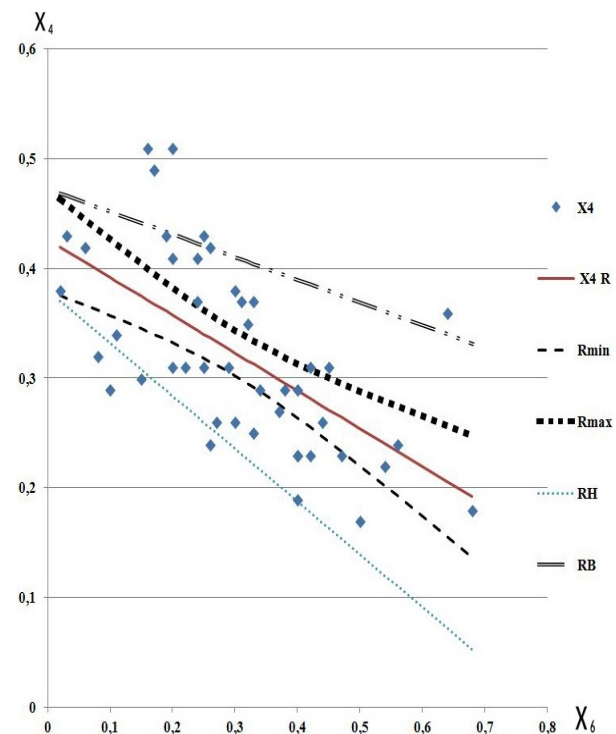
Рис. 2. Точечная и интервальная оценки регрессии X_4 на X_6 :
