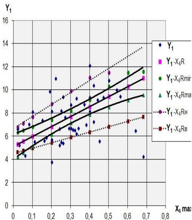
Рис. 3. Проверка адекватности модели
