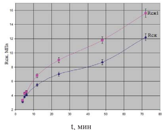
Рис. 1. Кривая изменения R_{сж} в процессе формирования структуры цементного камня: R_{сж} – не обработан, R_{сж I} – обработан в электромагнитном поле / Fig. 1. The curve of the change R_{сж} during the formation of the structure of cement stone: R_{сж} – not processed, R_{сж I} – processed in an electromagnetic field
