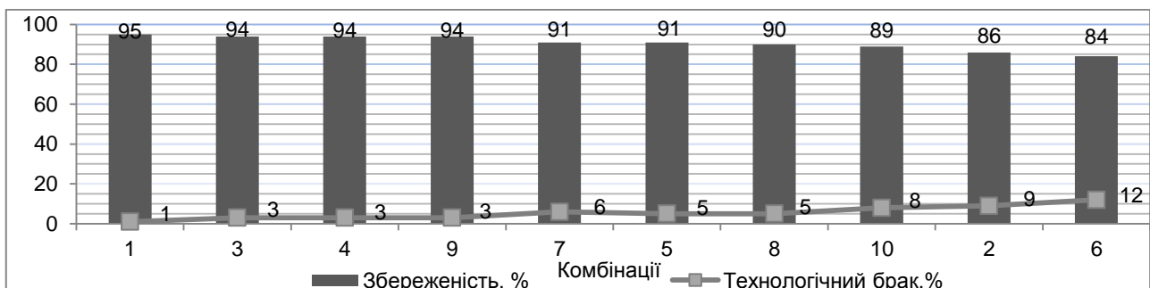
Рис. 4. Технологічний брак бульб потомства різних комбінацій (середнє за 2015-2016 рр.)
