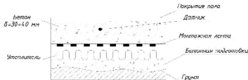
Рис.3. Пол в сухом помещении по грунту
