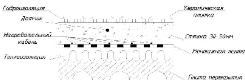
Рис.2. Пол в мокром помещении на перекрытии
