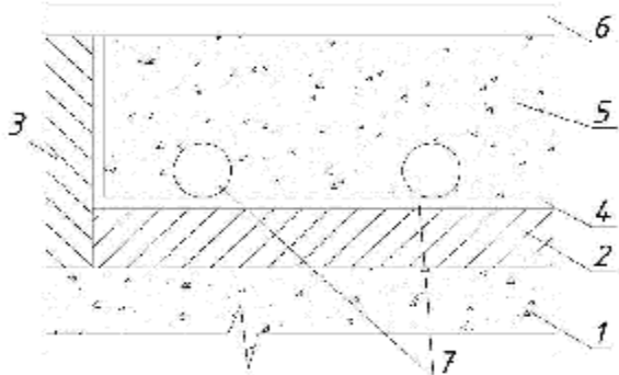
Рис. 8. Конструкция теплого пола
