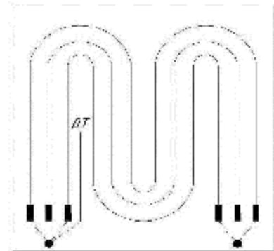
Рис.6 Три одножильные кабеля. Трехфазная система подключения по схеме звезда/треугольник ДТ- датчик температуры пола
