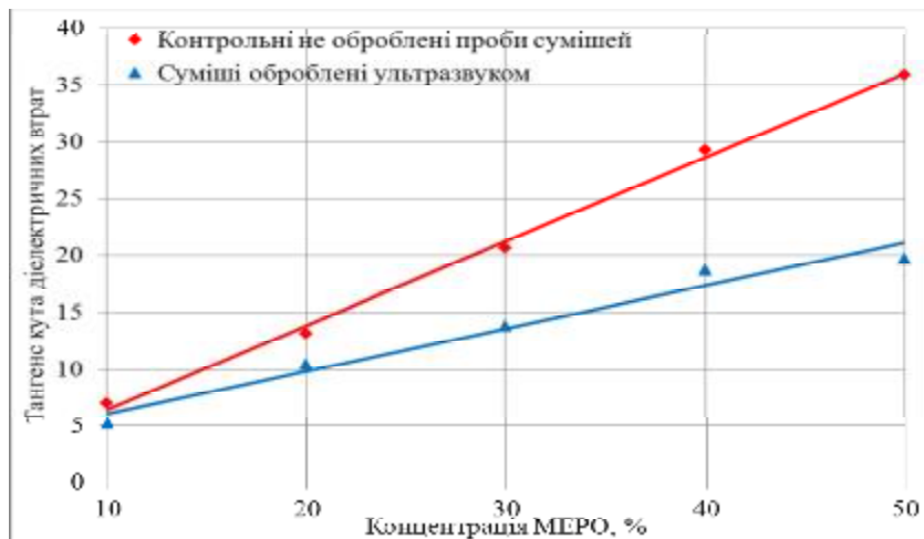
Рисунок 5 – Залежність тангенса кута діелектричних втрат від концентрації МЕРО в дизельному паливі до обробки і після обробки ультразвуковими хвилями
