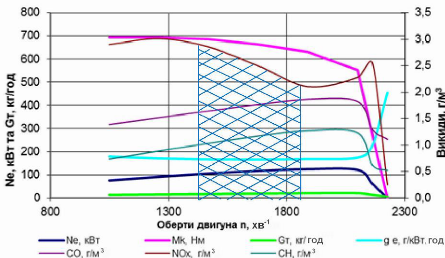
Рисунок 2 – Вплив режиму роботи двигуна ЯМЗ-236-М2 на загальну кількість викидів NOx, CO, CH. – оптимальний робочий діапазон трактора ХТЗ-170 з екологічної точки зору.
