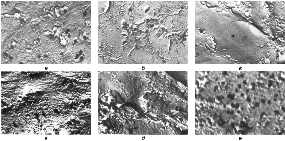
Рис. 2. Нанорозмірні нітриди ванадію (чорні включення) в поліпшених сталях 20ХГСАФЛ (а), 40ХГСАФЛ (б), 20ХГЗСАФЛ (в), 20ХГЗСАФЛ (г), 20ХЗГСАФЛ (д) і армко-залізі (е): а, б в, г, д - збільшення 27000; е - 39000.
