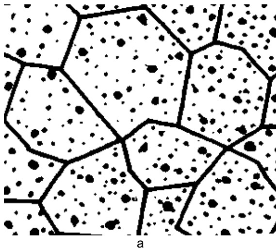
Рис. 1. Дисперсна (а) і агрегатна (б) структура дисперсійно - твердих сплавів
