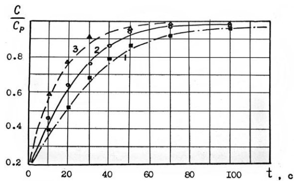
Рис. 3 Кінетика вимивання забруднень з супіщаного ґрунту
