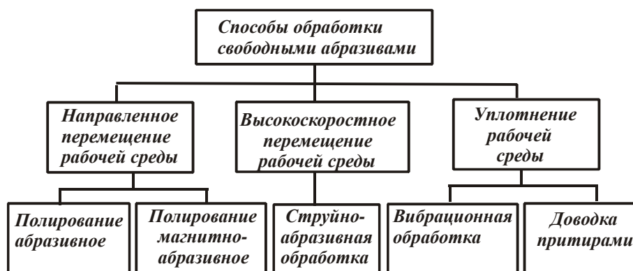
Рисунок 1 – Классификация способов обработки свободными абразивами по характеру воздействия абразивной частицы
