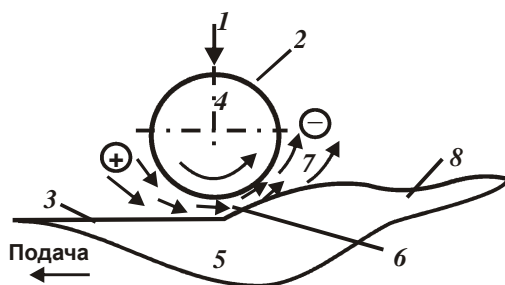
Рисунок 2 – Схема полирования суспензией на основе ультрадисперсного порошка
