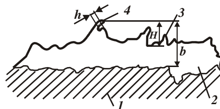
Рисунок 5 – Параметры граничного слоя металлической поверхности: 1 – деталь; 2 – неметаллическая пленка; 3 – микронеровность; 4 – субмикронеровность; h и H – высоты соответственно микронеровности и субмикронеровности; b – средняя толщина неметаллической пленки.
