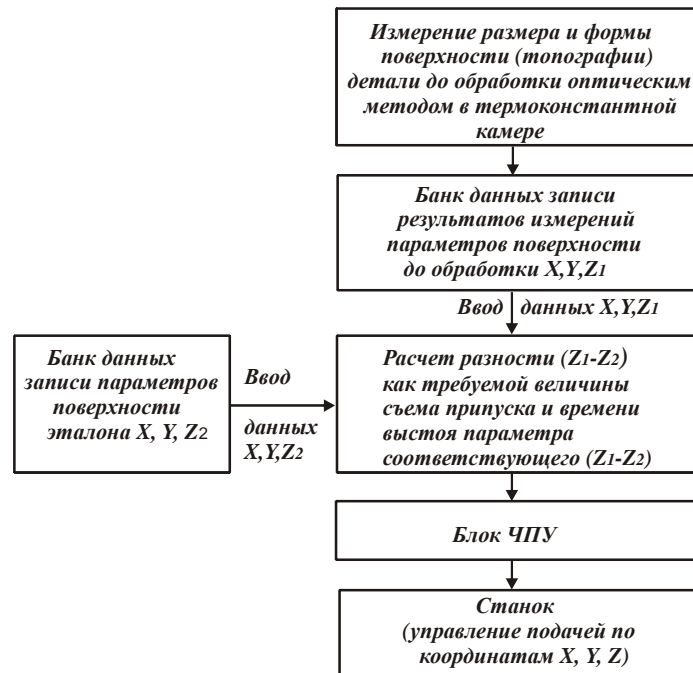
Рисунок 3 – Схема управления процессом формообразования поверхностных слоев деталей
