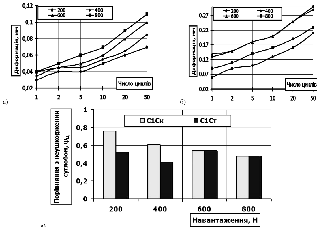
Рисунок 5 – Залежності залишкової деформації непошкоджених суглобів (а) та систем ССк (б) від числа циклів навантаження; співвідношення залишкових деформацій неушкоджених суглобів та препаратів з фіксованими переломами за 50 циклів навантаження \psi_u = \Delta^H / \Delta^C_{50} (в)
