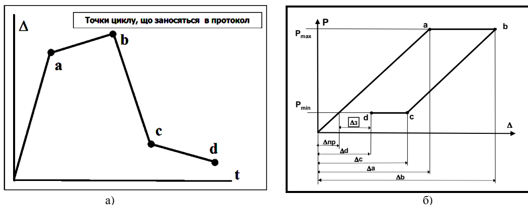
Рисунок 4 – Схематизація кривої "час – деформація" (а) та схема циклу у координатах "навантаження – деформація" (б)
