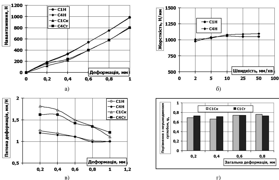
Рисунок 3 – Діаграми деформування суглобів при стискуванні (а), залежності жорсткості суглобів від швидкостей деформування (б), зміна приведених деформацій при зростанні загальної деформації (в) та порівняння неушкоджених та пошкоджених суглобів (г)
