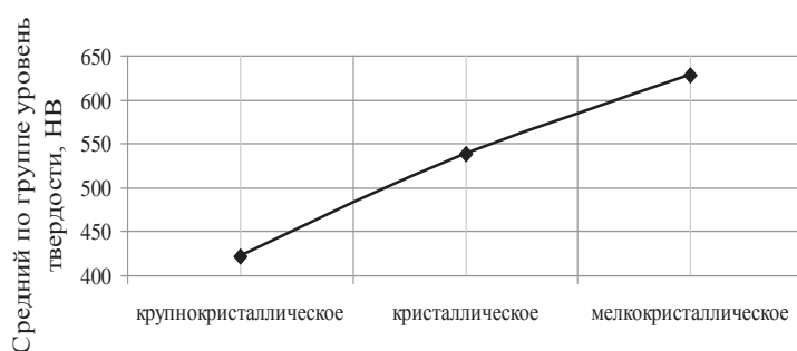
Рис. 1. Зависимость уровня прочности от строения излома образца
