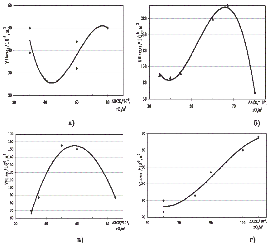
Рис. 2 Залежність виділення біогазу ( V біогазу, m^3 ) від зміни показника ХСК ( \Delta XSK , гO_2/m^3 ) при деструкції активного мулу: а) контроль; б) при хімічній дезінтеграції; в) при механічній дезінтеграції; г) при термічній дезінтеграції.
