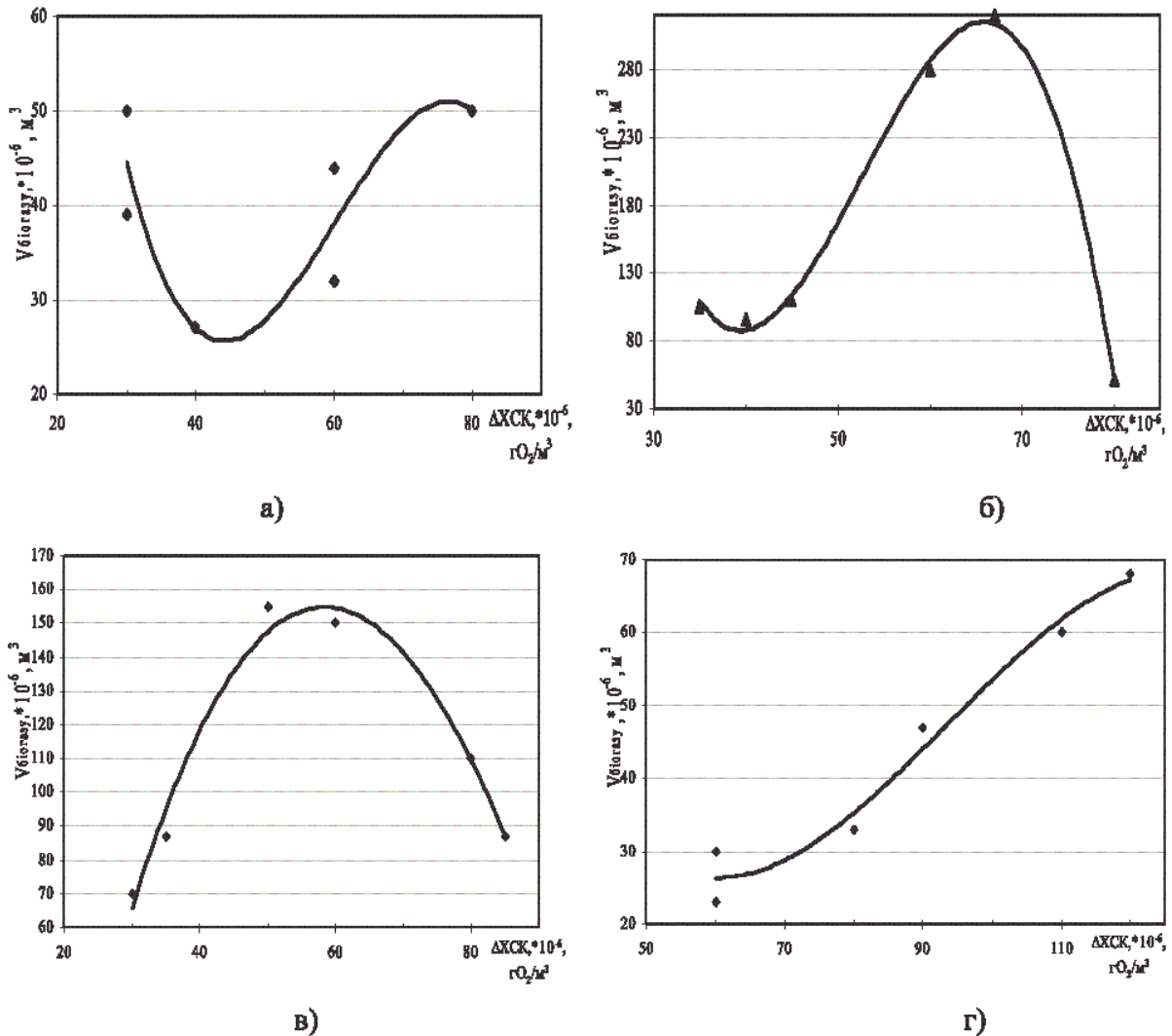
Рис. 2 Залежність виділення біогазу ( V біогазу, \text{м}^3 ) від зміни показника ХСК ( \Delta\text{ХСК} , \text{гO}_2/\text{м}^3 ) при деструкції активного мулу: а) контроль; б) при хімічній дезінтеграції; в) при механічній дезінтеграції; г) при термічній дезінтеграції.
