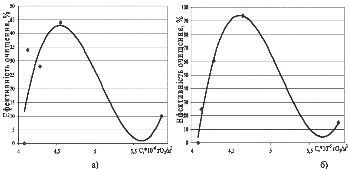
Рис.1 Динаміка зміни концентрації забруднюючих речовин від концентрації розчиненого кисню ( C, \text{гO}_2/\text{м}^3 ) у біореакторі: а) за азотом; б) за фосфатами.
