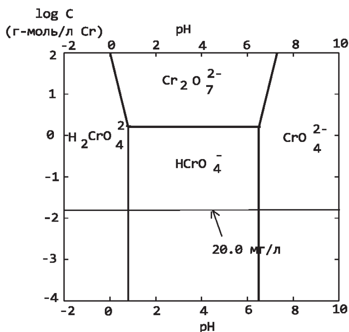
Рис. 4. Диаграмма состояния ионных форм Cr (VI) в водных растворах.
