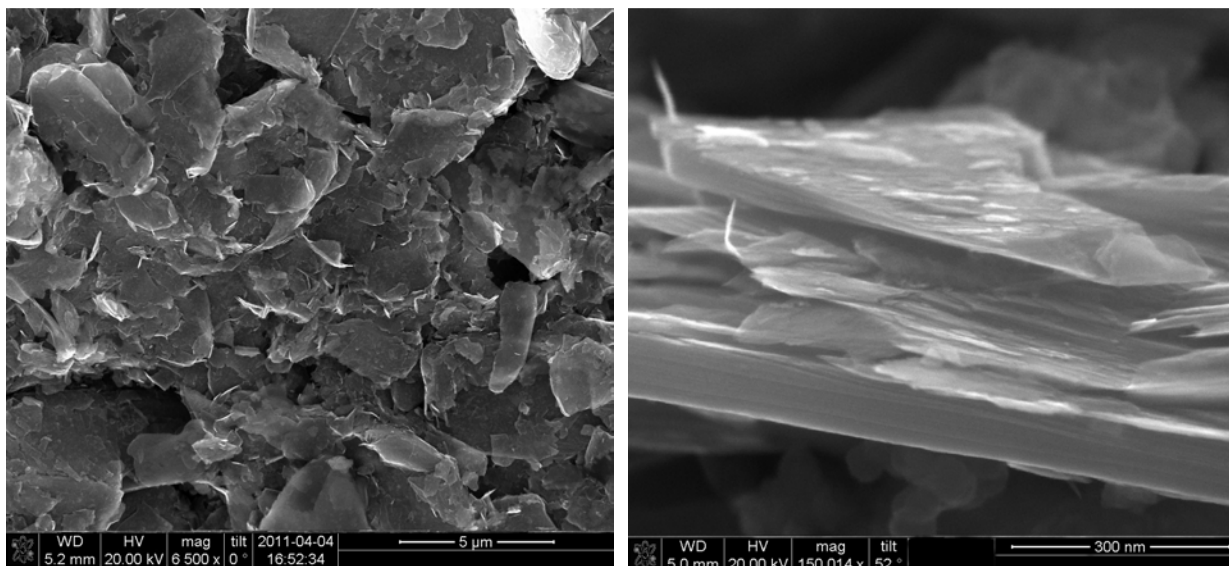
Рис. 2. СЕМ мікрознімки отриманих НПГ
