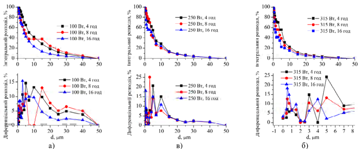
Рис. 3. Розподіл частинок НПГ після обробки ультразвуком за різних параметрах (час, потужність)
