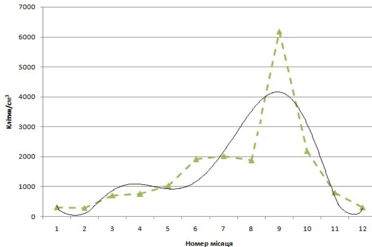
Рис. 4. Апроксимація процесів розвитку зелених водоростей (середнє значення для двох водосховищ): штрихова лінія – дані експериментальних досліджень; суцільна лінія – апроксимація експериментальних даних поліномом 6-го ступеня
