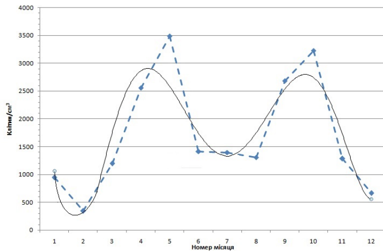
Рис. 2. Апроксимація процесів розвитку діатомових водоростей (середнє значення для двох водосховищ): штрихова лінія – дані експериментальних досліджень; суцільна лінія – апроксимація експериментальних даних поліномом 5-го ступеня
