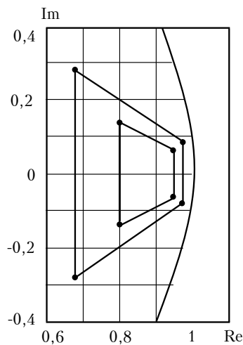
Рис. 2. Ділянка z площини для визначення коренів характеристичного рівняння
