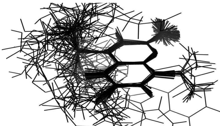
Рис. 3. Просторові конформації досліджених структур (стрижнева модель відображення)
