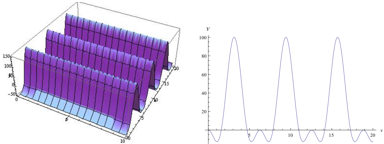
Рис. 4. Поведінка потенціальної функції системи з параметрами, не залежними від часу при заданому значенні параметра управління \mu = 1
