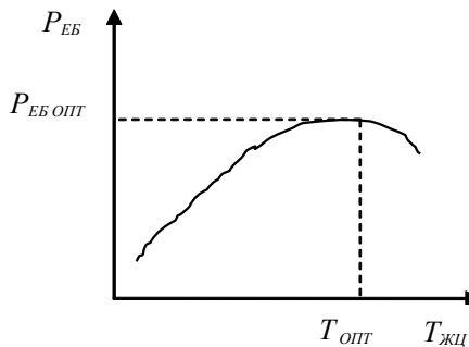
Рис. 5. Графічна інтерпретація залежності P_{ЕБ} ( T_{жц} )
