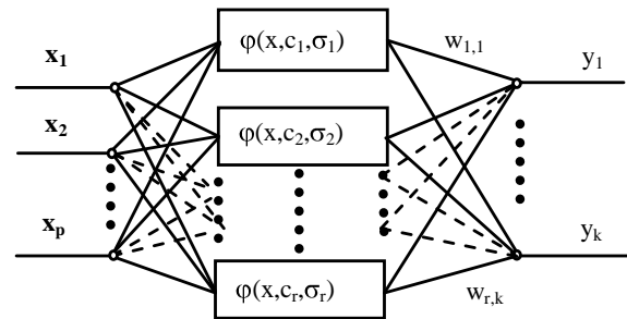
Рис. 1. Архітектура p-r-k РБФ-мережі
