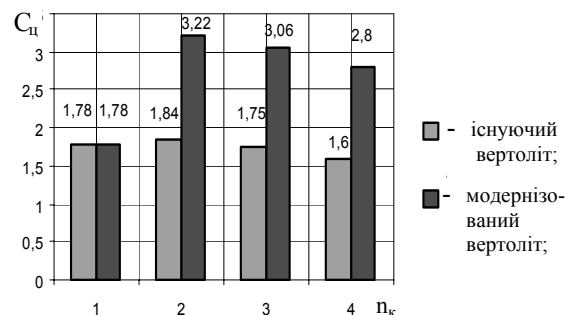
Рис. 4. Залежність нанесеного збитку груповій цілі від кількості каналів в вертольоті
