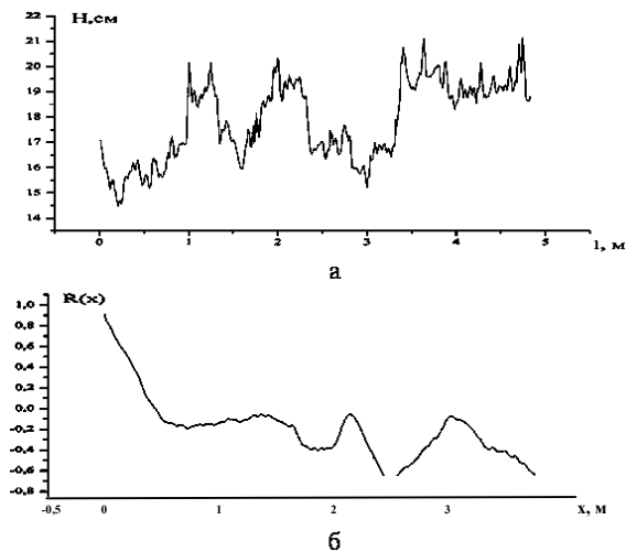
Рис. 3. Профилограмма а – засеянного свеклой поля и б – ее автокорреляционная функция
