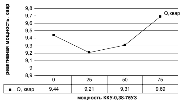
Рис. 7. График зависимости мощности компенсирующих устройств \text{РККУ} = f(Q)
