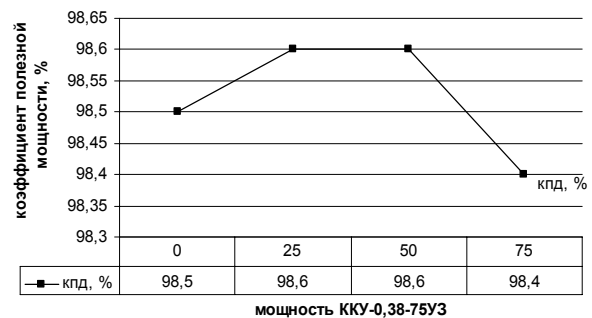
Рис. 6. График зависимости мощности компенсирующих устройств \text{РККУ} = f(\eta)
