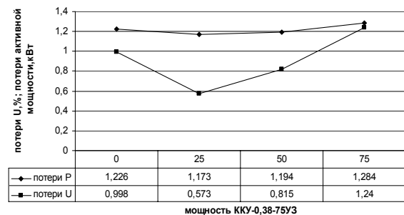
Рис. 5. График зависимости мощности компенсирующих устройств \text{РККУ} = f(\Delta P, \Delta U)
