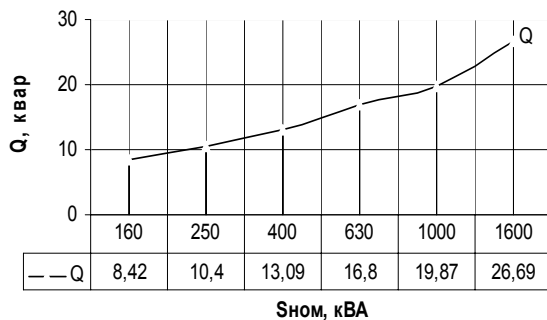
Рис. 3. График зависимости мощности трансформаторов S_{ном} = f(Q)
